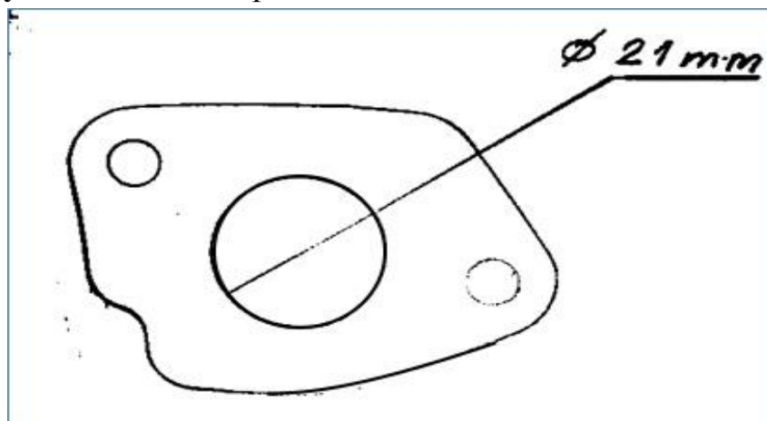
Рисунок 5 – эскиз ограничительной шайбы
