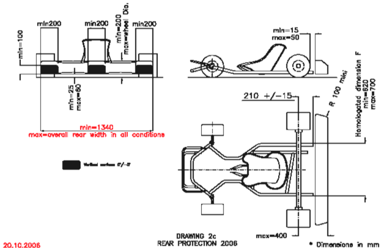
Рисунок 2 – задний пластиковый отбойник СИК FIA
