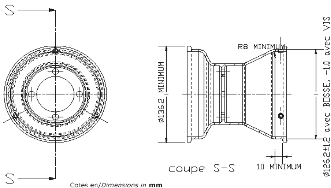
Рисунок 4 – эскиз колесного диска
