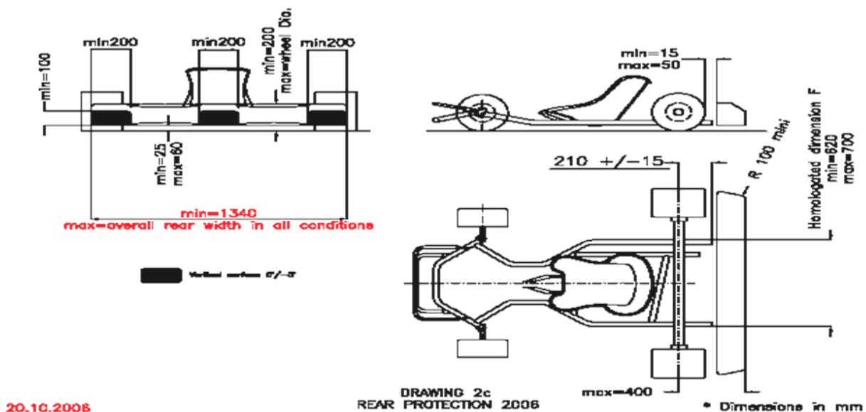
Рисунок 2 – задний пластиковый отбойник СИК FIA
