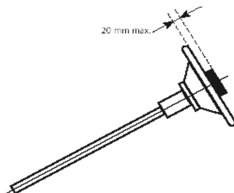
Рисунок 3 – установка приборов на рулевом колесе
